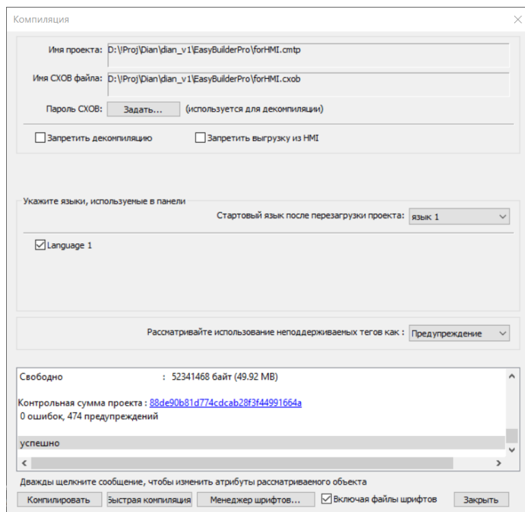
Рисунок 2.3 – Окно «Компиляция»
