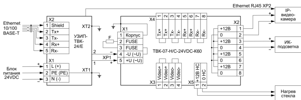
г) Подключение термокожуха на примере модификации ТБК-07-С-24VDC-K60 с устройством защиты УЗИП-ТБК-24/Е и IP-видеокамерой
