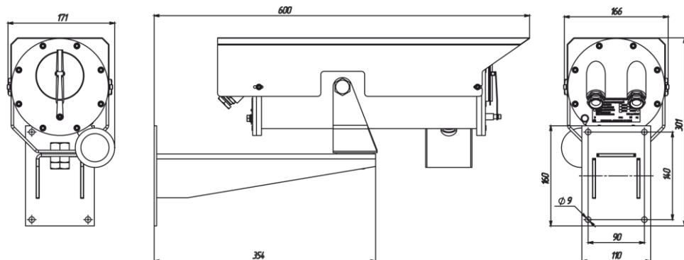
в) Внешний вид термокожуха ТВК-07-Н/С-И1 с модулем ИК подсветки (ИКХХХ, опция) и очистки стекла (W, опция)
