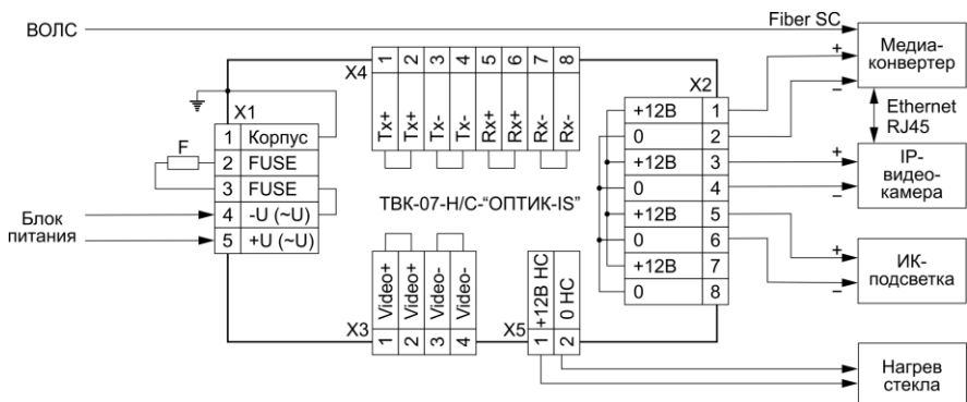
б) Подключение термокожуха на примере модификации TBK-07-Н "ОПТИК-IS"-K60 с ИК-подсветкой, IP-видеокамерой и медиаконвертером
