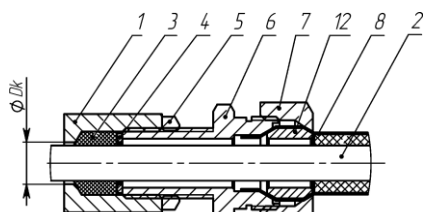
а) монтаж бронированным кабелем в кабельном вводе КВБ17
