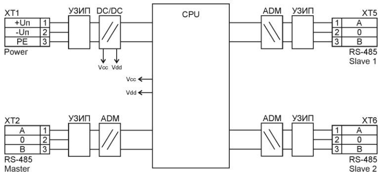
Рисунок 3 – Структурная схема MC-11
