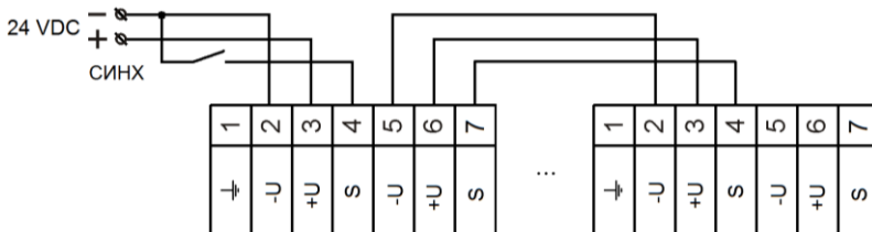
Рисунок 5. Внутренняя схема контроля цепи оповещателей BC-07e-Eх-3(И)-24VDC.
