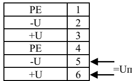
б) BC-07e-СД-24VDC
