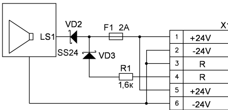
а) BC-07e-Eх-3-24VDC
