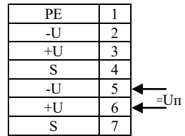
в) BC-07e-СЛ-24VDC
